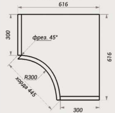
Нижний модуль
