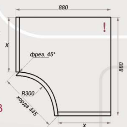
Нижний модуль
