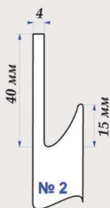
сквозная №2
