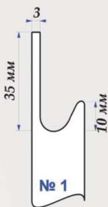
сквозная №1
