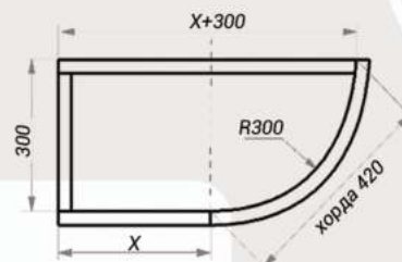
Нижний модуль
